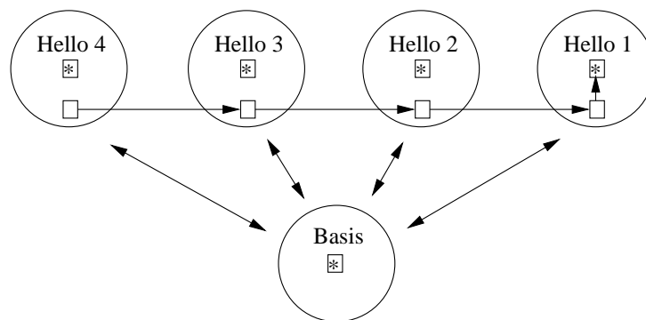
Abbildung 1: Die für Aufgabe 2 gewünschte Verkettung.
